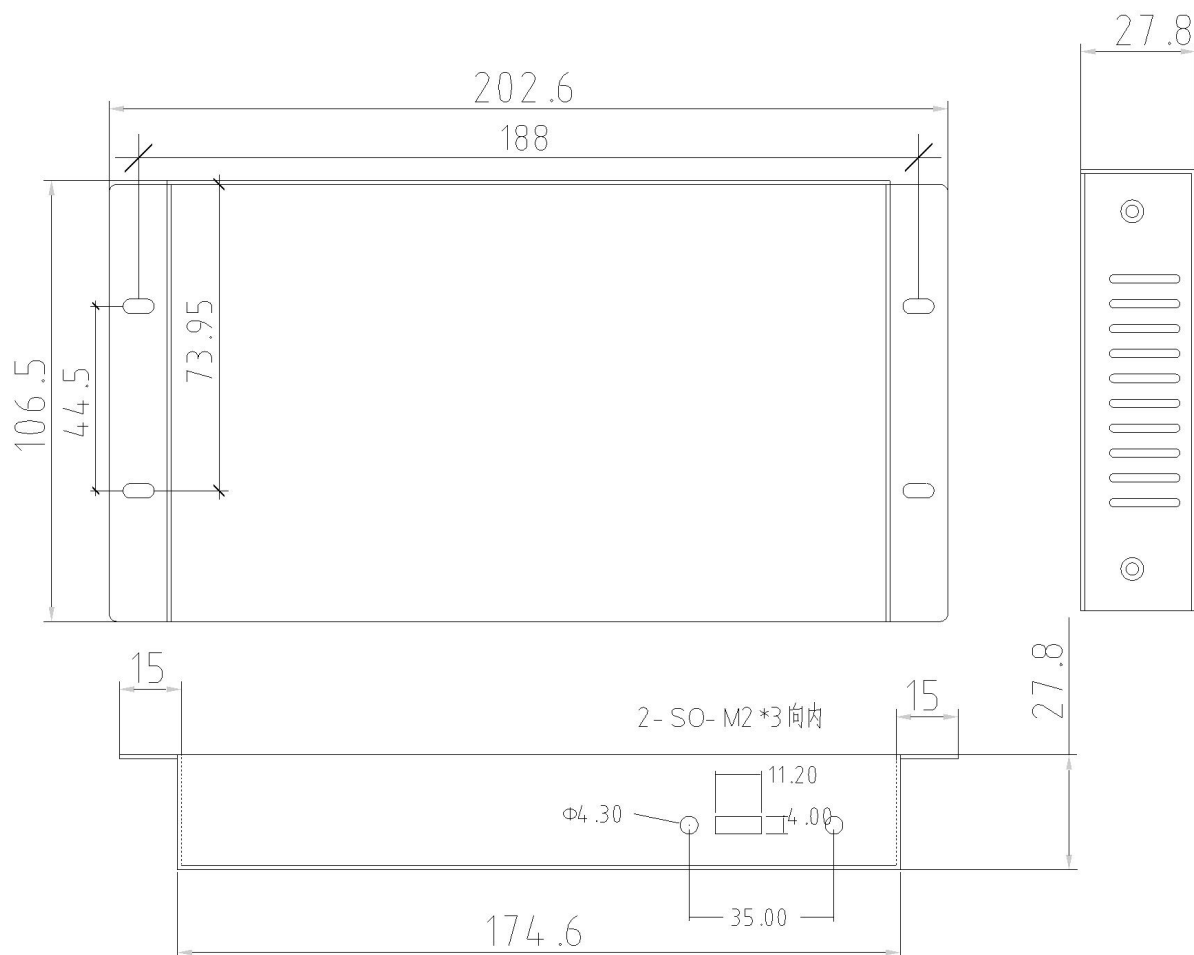
側面接口尺寸 (裝盒)
